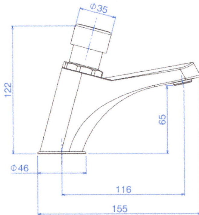
Desenho Técnico
